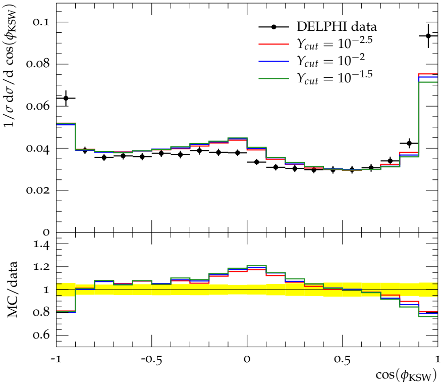
Körner-Schierholz-Willrodt \cos(\phi_{\text{KSW}}) , Durham y_{\text{cut}} = 0.008
